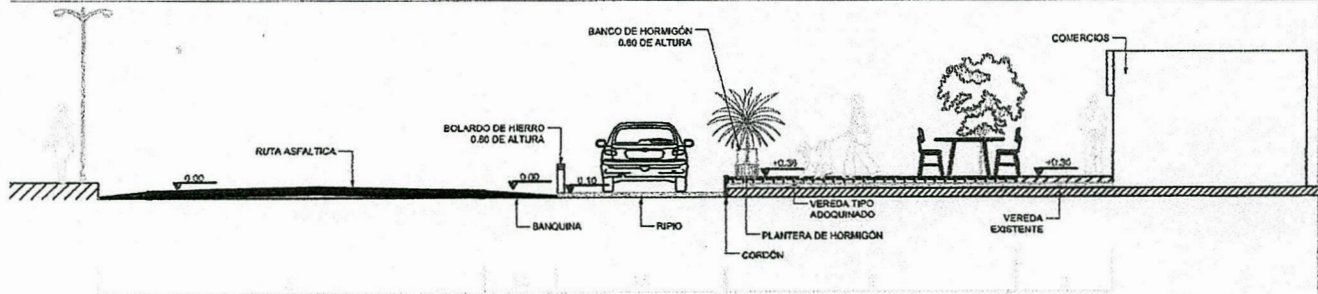
PERFIL DE CALLE
