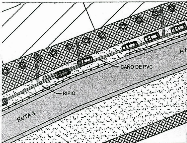
PLANTA DE DESAGÜE
