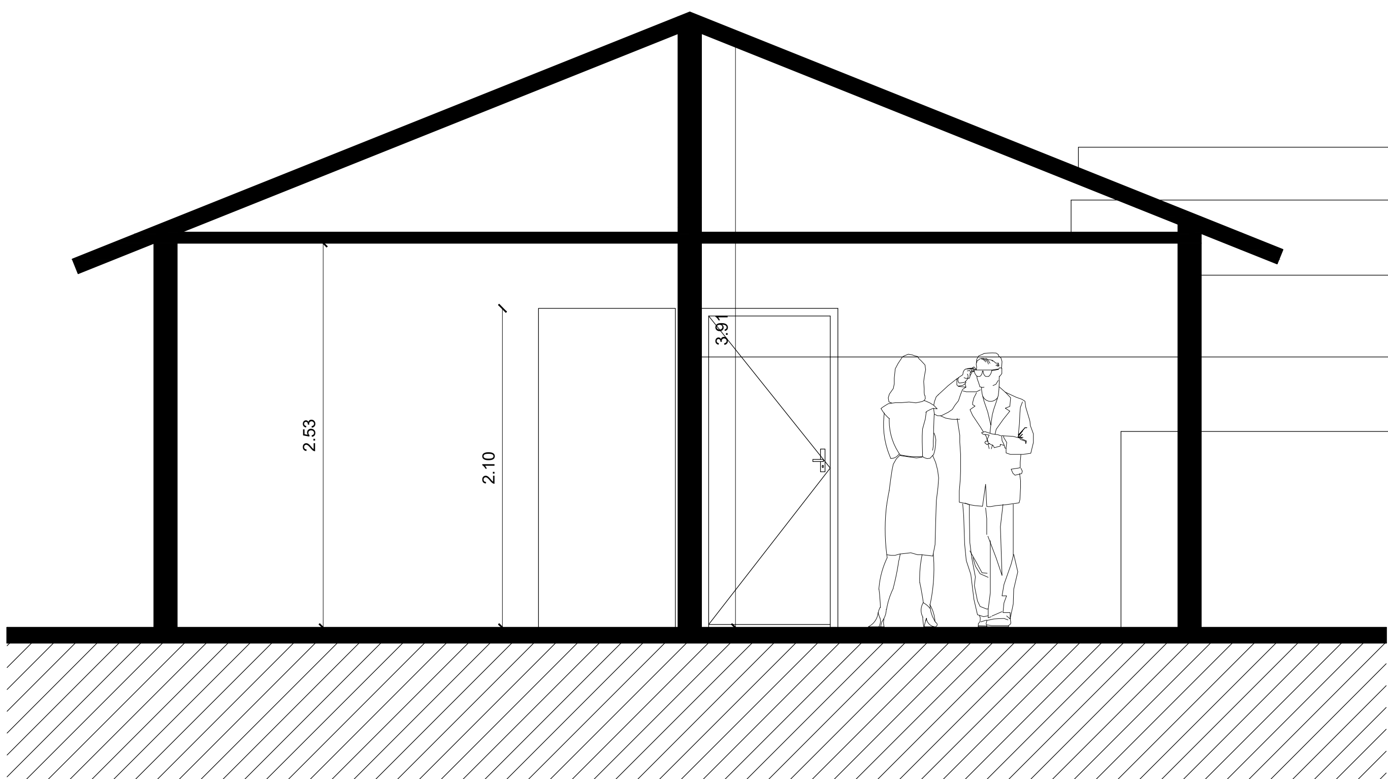
CORTE TRANSVERSAL A-A' ESCALA -----1:50
