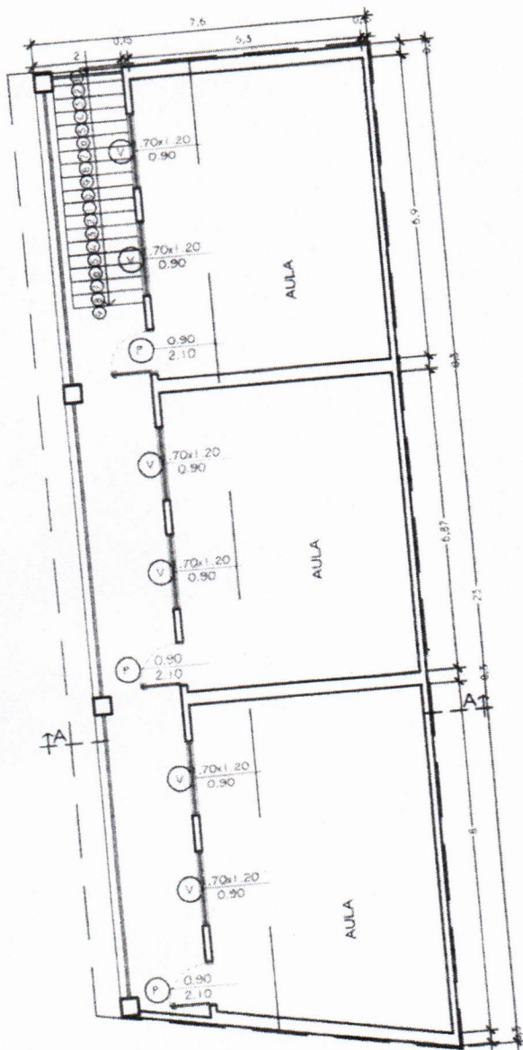
PLANTA ARQUITECTONICA Esc.: 1/75
