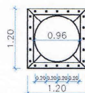
CORTE I-I
