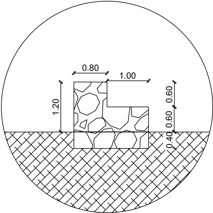
CORTE LATERAL
