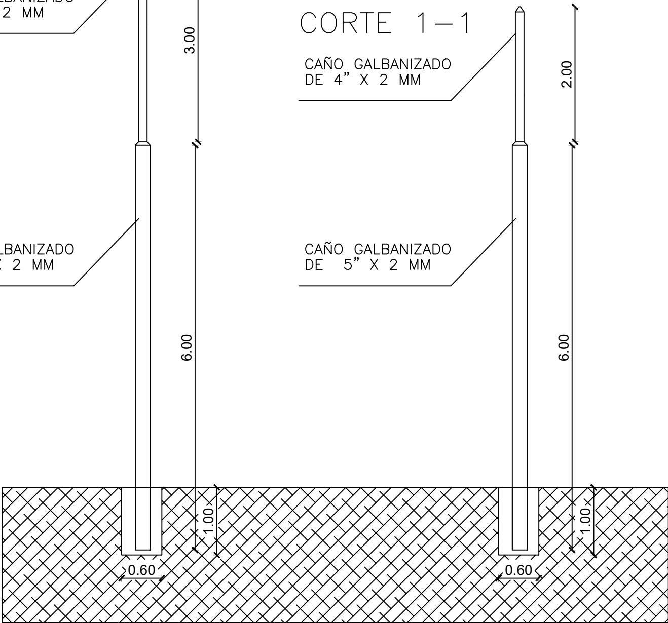
CORTE 1-1
