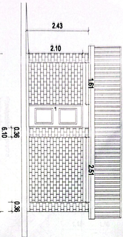
FACHADA FRONTAL
