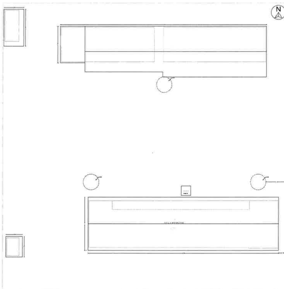
Planta de Techo Escala 1.500
