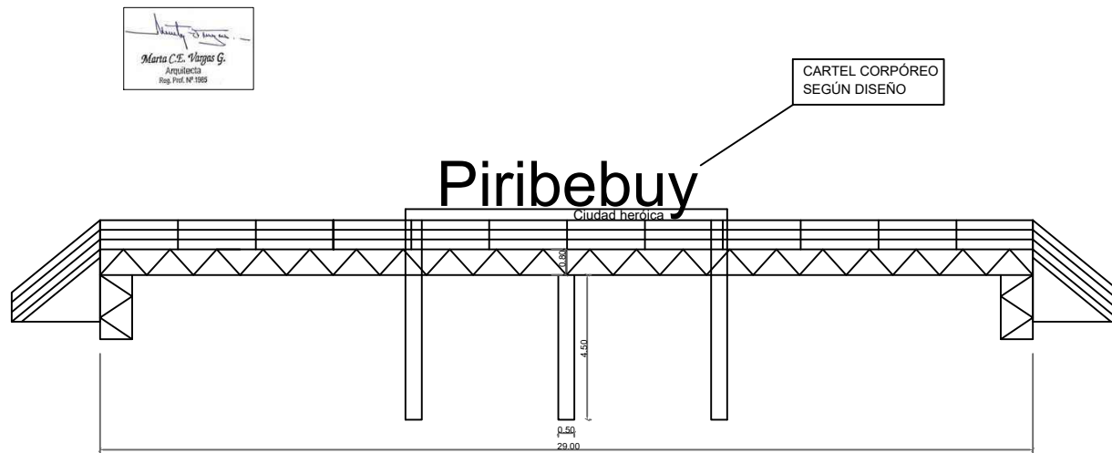
ALZADO
