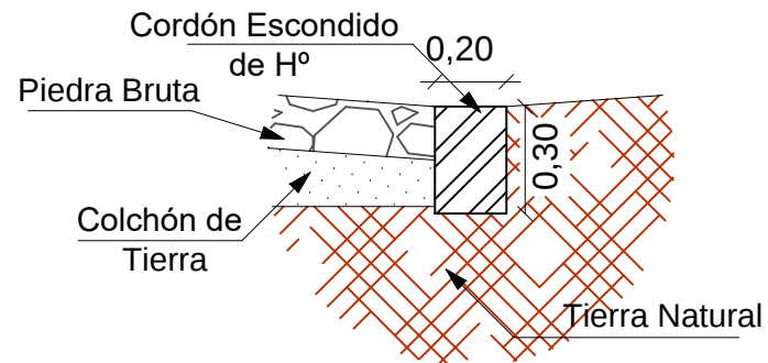
DETALLE DE CORDÓN BOCA CALLE Esc: 1__30
