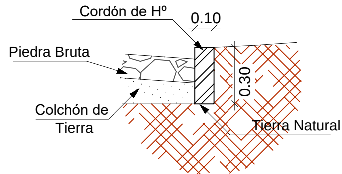
DETALLE DE CORDÓN BOCA CALLE Esc: 1__30
