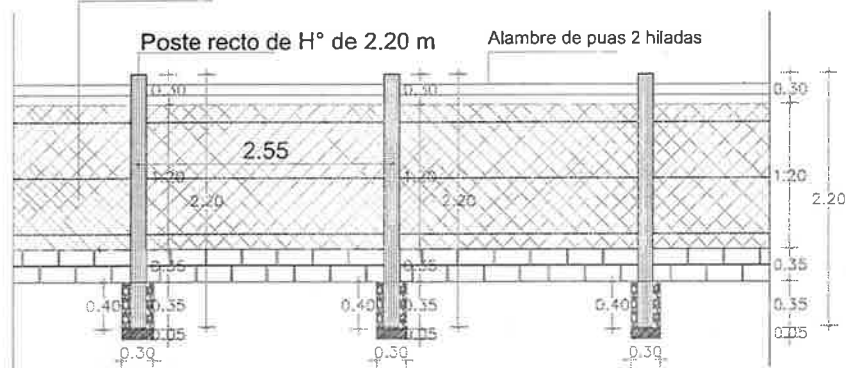
DETALLE DE CERCADO Esc: 1/75
