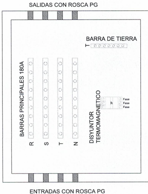
MODELO DE TABLERO PRINCIPAL
