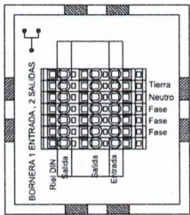
MODELO DE CAJA DE DERIVACIÓN
