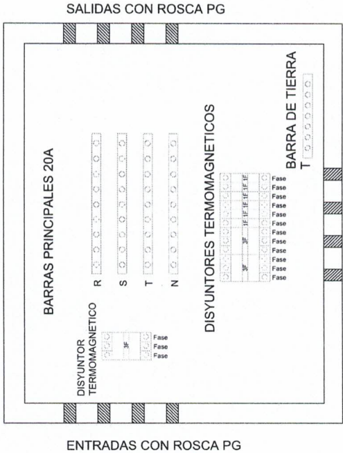
MODELO DE TABLERO DE CONTROL /LUCES EXT / ADMINISTRACION
