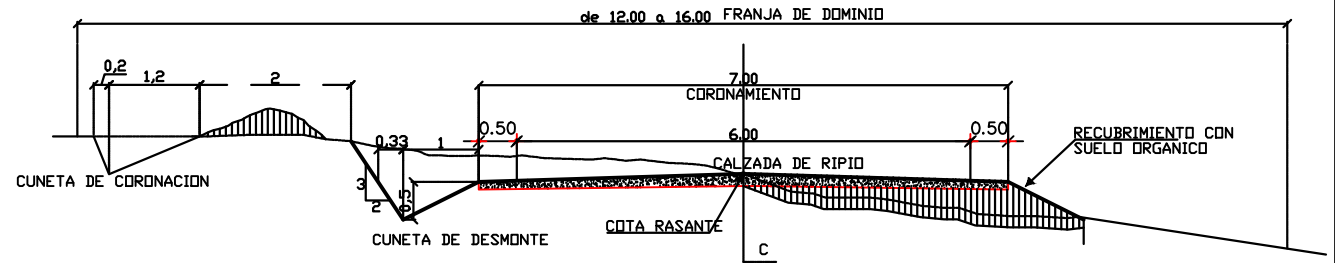
SECCION EN MEDIA LADERA ESC.-----1/50
