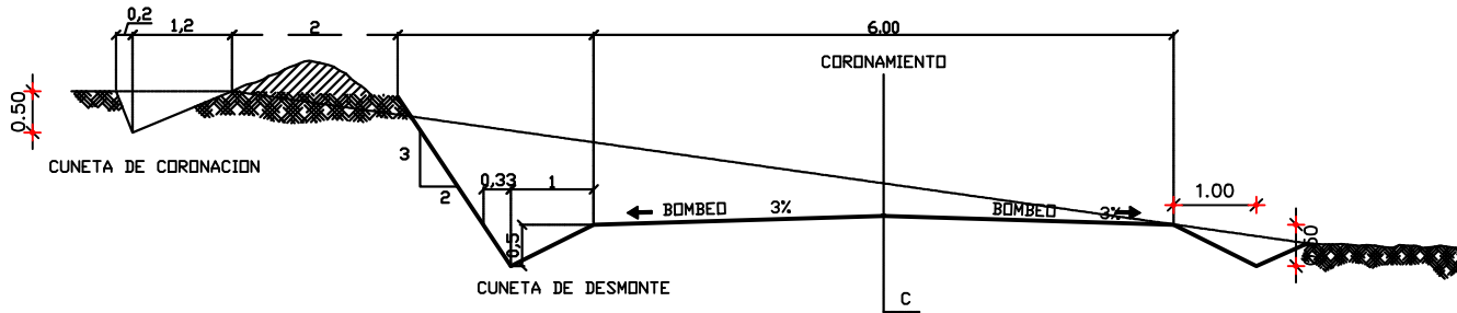
SECCION DE DESMONTE ESC.-----1/50
