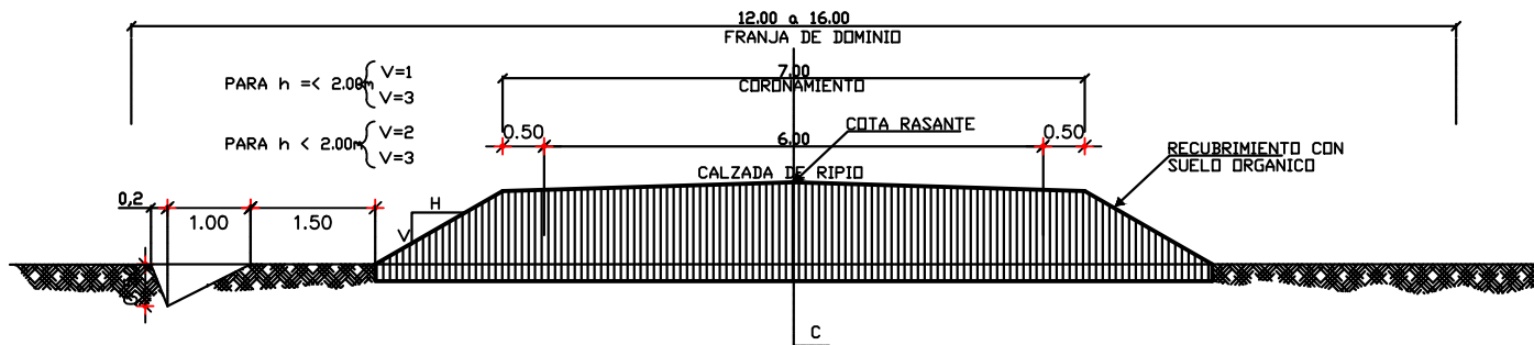
SECCION EN TERRAPLEN ESC.-----1/50
