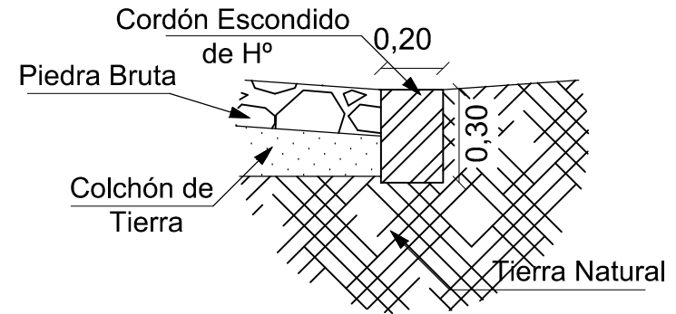
DETALLE DE CORDÓN BOCA CALLE Esc: 1__30
