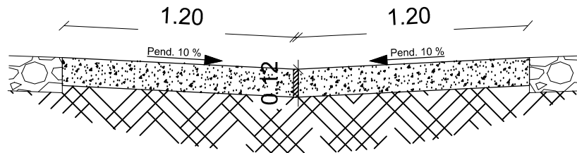
DETALLE BADEN DE H° Esc: 1__20
