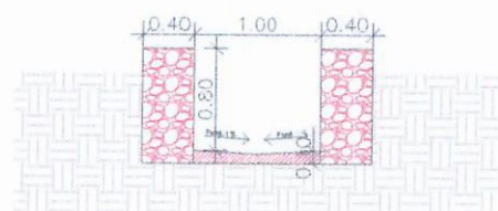
DETALLE DE CANAL A CIELO ABIERTO
