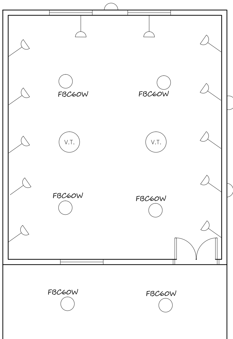
Esquema eléctrico Esc.1/100
