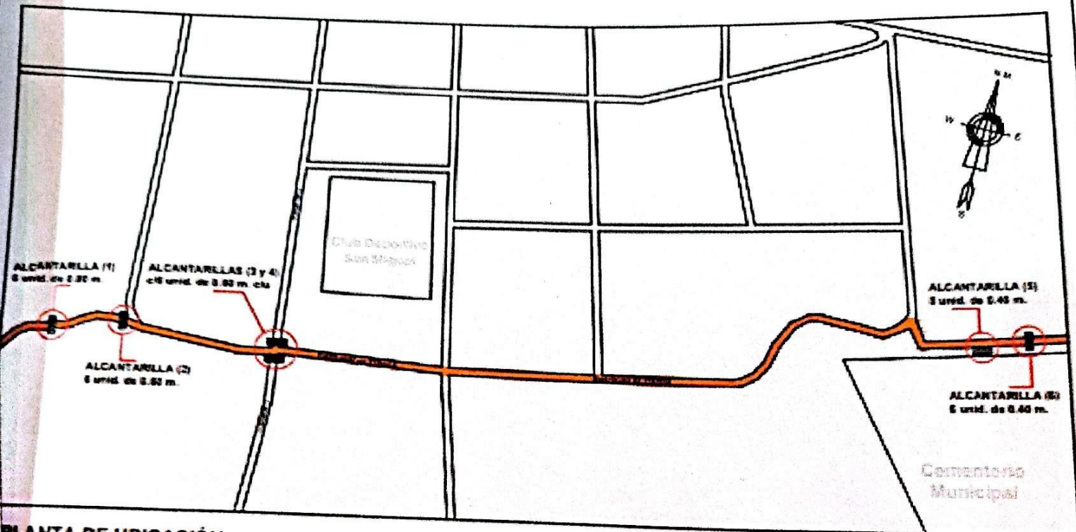
PLANTA DE UBICACIÓN
