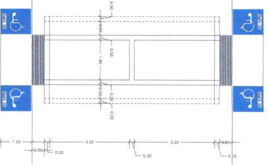
DETALLE DE VIGA
