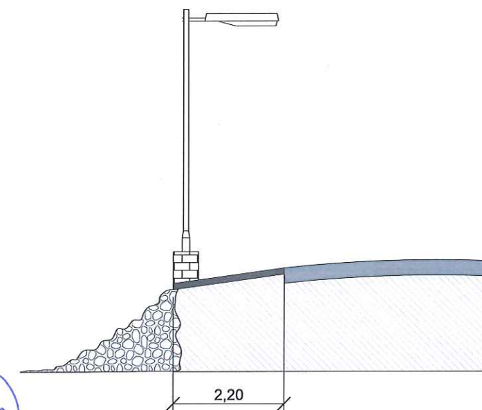
SECCIÓN F-F Esc. 1:100
