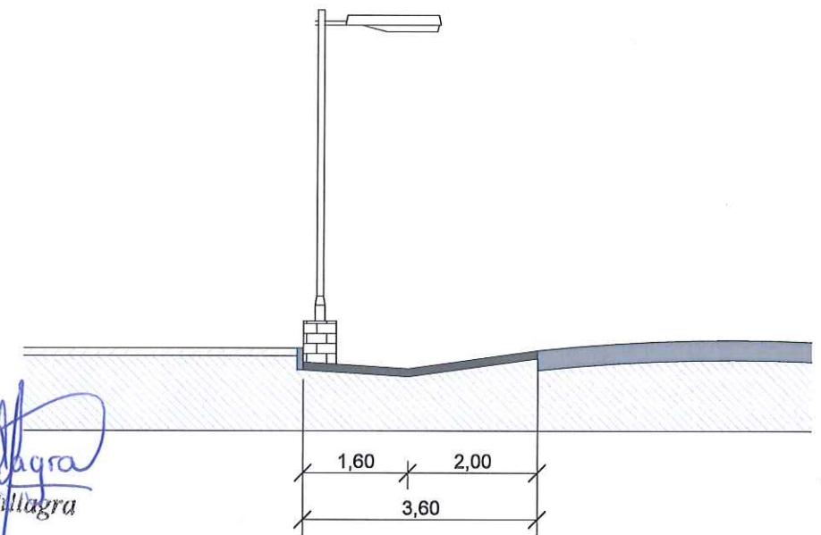
SECCIÓN B-B Esc. 1:75
