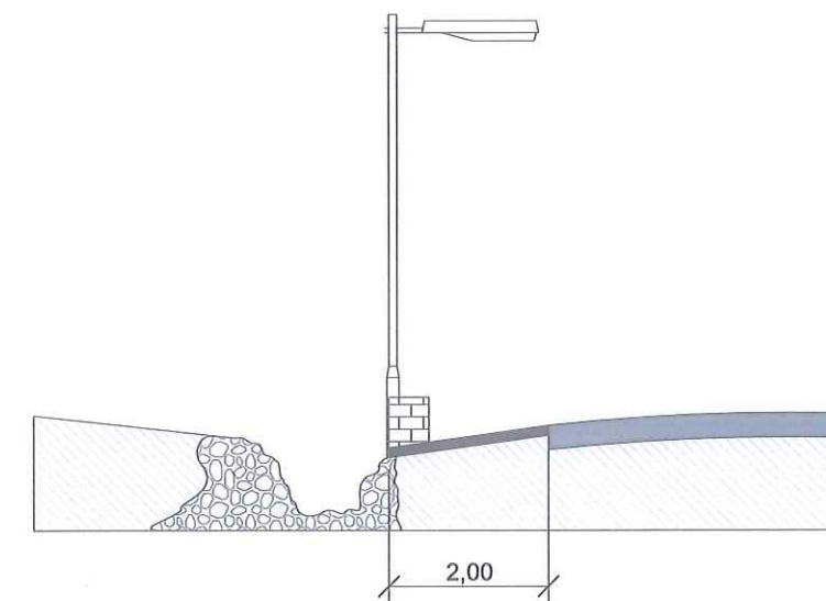
SECCIÓN E-E Esc. 1:100
