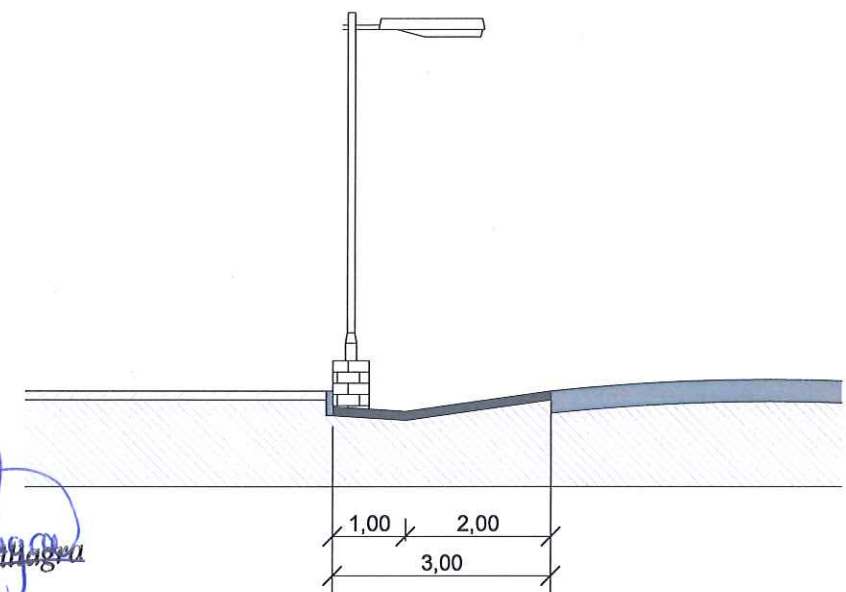
SECCIÓN D-D Esc. 1:100
