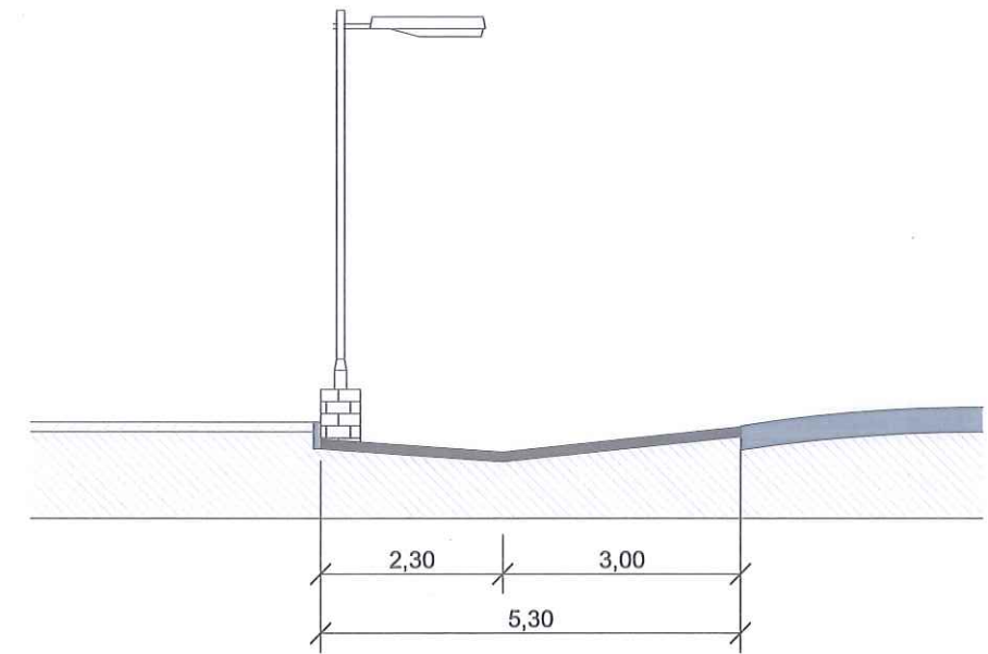
SECCIÓN C-C Esc. 1:100
