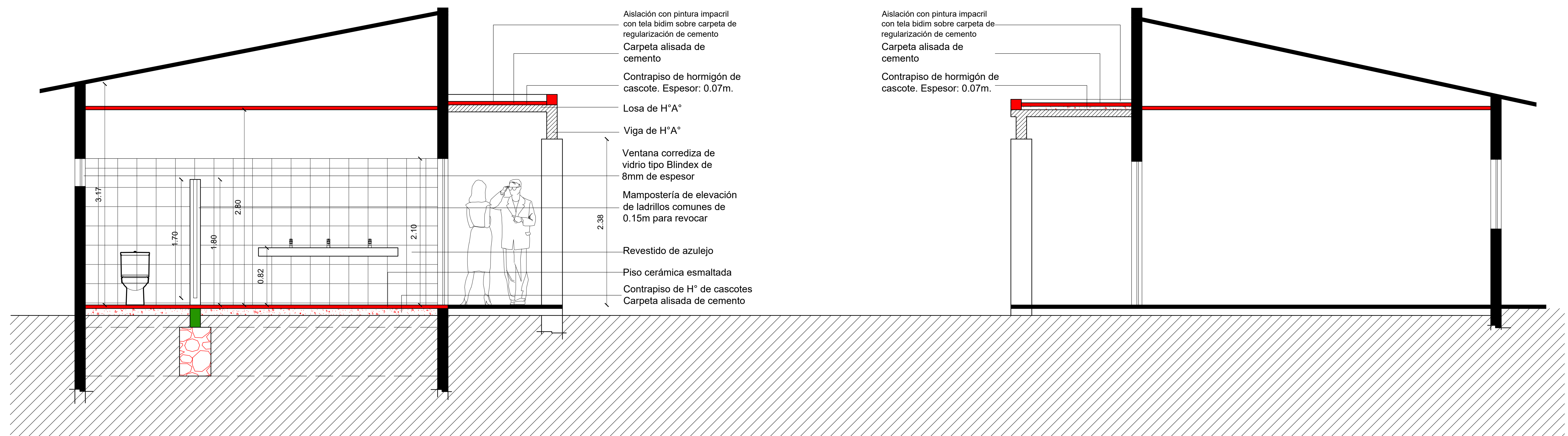
CORTE TRANSVERSAL A-A' ESCALA -----1:50
