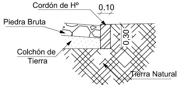
DETALLE DE CORDÓN SIMPLE Esc: 1__30
