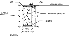
DETALLE VIGA CORDÓN HoAo ESC.....1/25
