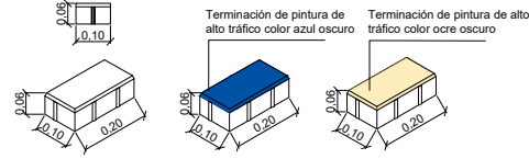
DETALLE PISO ADOQUIN RECTANGULAR DE CONCRETO ECOLÓGICO 6X10X20 ESC.....1/15
