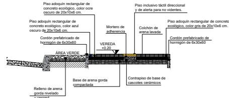
DETALLE VEREDA CON ÁREA VERDE ESC.....1/50
