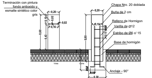
DETALLE BOLARDO DE HORMIGÓN ESC.....1/25
