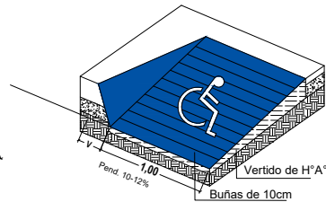
DETALLE RAMPA PEATONAL ESC.....1/50
