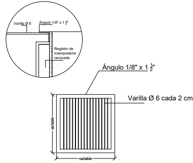
DETALLE PISO INCLUSIVO TÁCTIL DIRECCIONAL Y DE ALERTA ESC.....1/25
