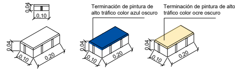
DETALLE PISO ADOQUIN RECTANGULAR DE CONCRETO ECOLÓGICO 4X10X20 ESC.....1/15
