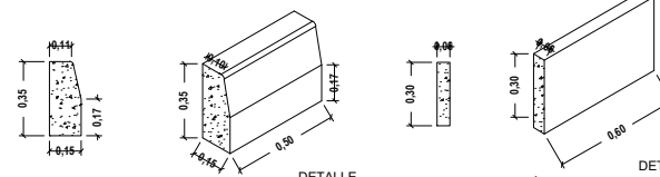
DETALLE CORDÓN PREFABRICADO DE H° 11X35X50 CM ESC.....1/25
