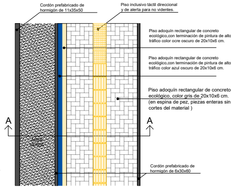
DETALLE PISO DE VEREDA ESC.....1/50
