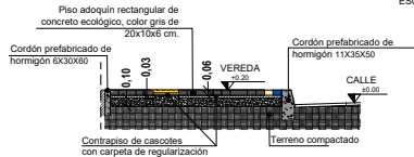
CORTE A-A ADOQUÍN SOBRE CONTRAPISO Y CARPETA
