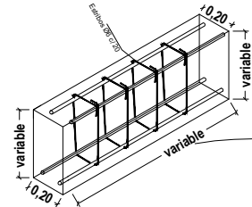
ISOMETRÍA CON DIMENSIONES
