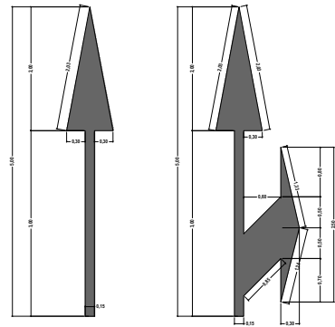
DETALLE PINTURA TERMOPLÁSTICA PARA SEÑALIZACIÓN DE SENTIDO DE CALLES (APLICACIÓN EN CALIENTE) ESC.....1/50
