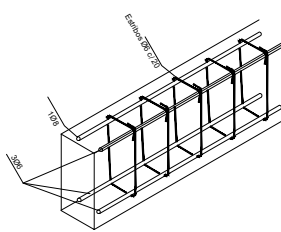
ISOMETRÍA CON DETALLES
