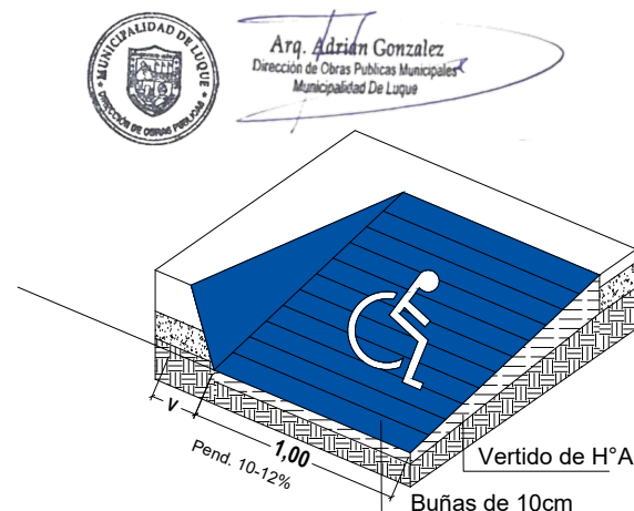
DETALLE RAMPA PEATONAL ESC.....1/50
