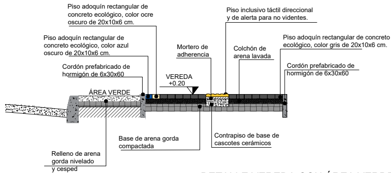
DETALLE PISO DE VEREDA ESC.....1/50
