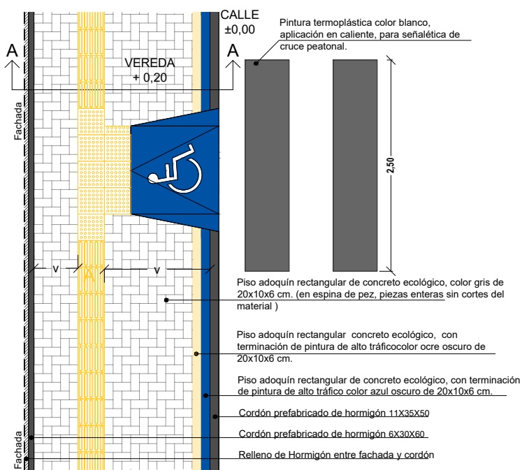
DETALLE PISO DE VEREDA ESC.....1/50
