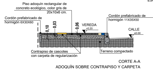
DETALLE PISO DE VEREDA ESC.....1/50
