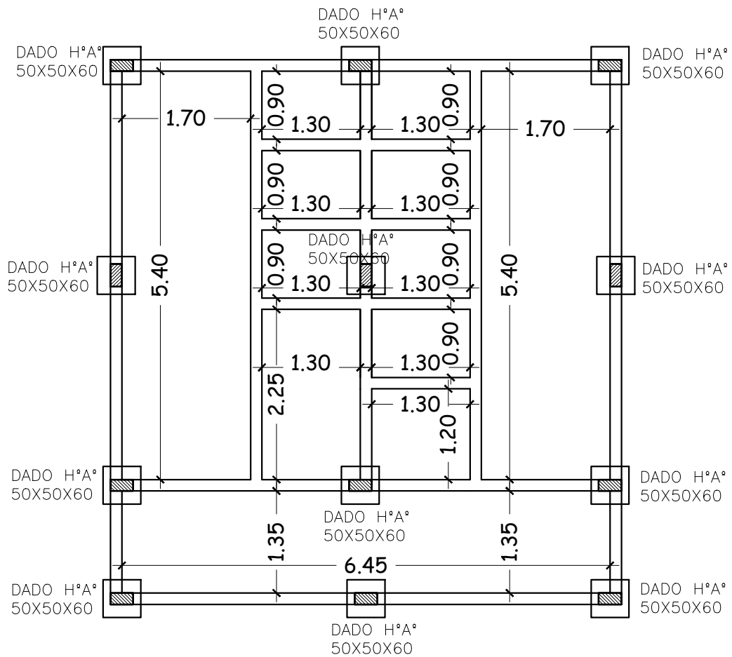
PLANTA DE FUNDACION
