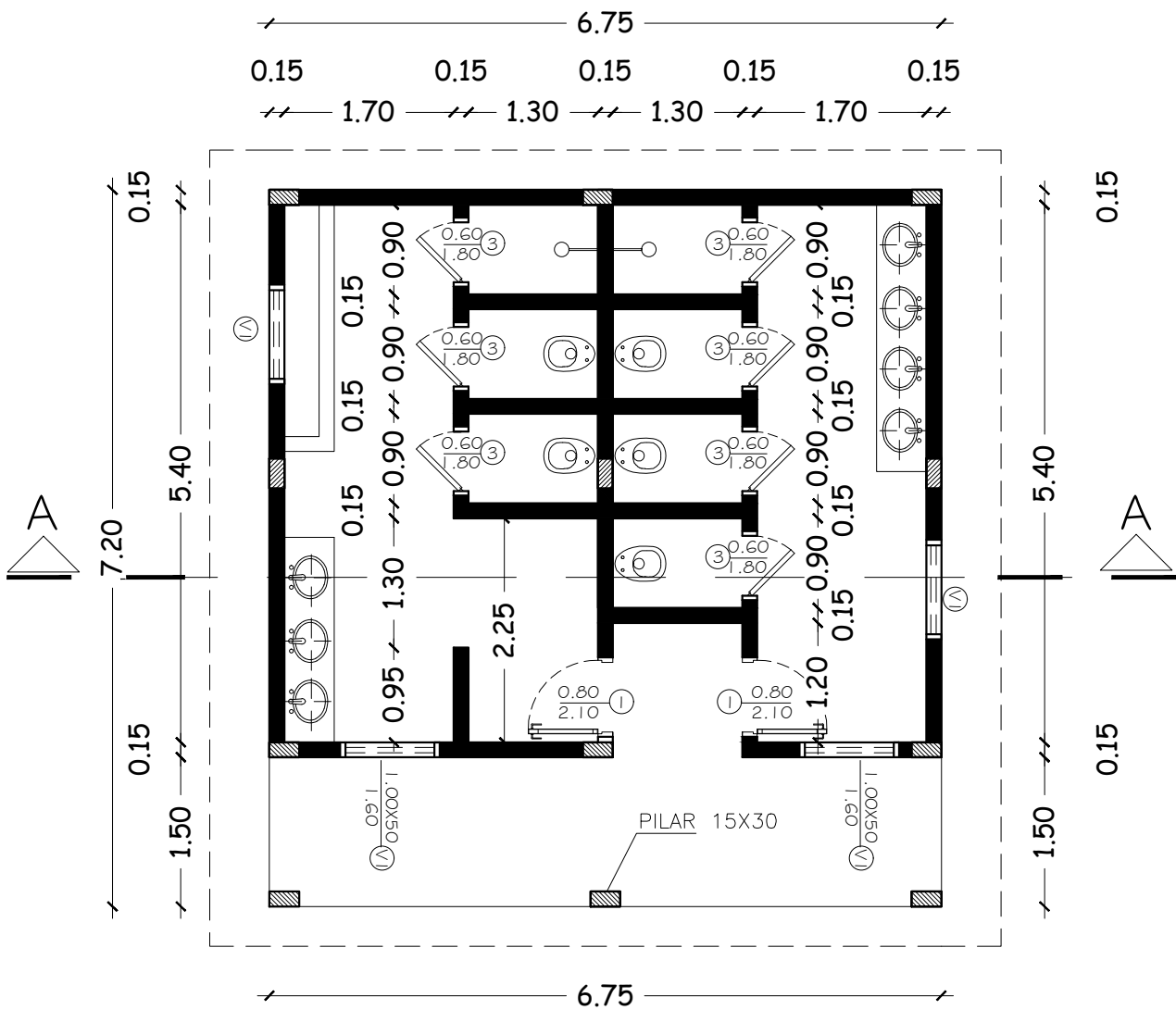
PLANTA ARQUITECTONICA
