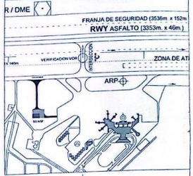
PLANO DE IMPLANTACIÓN BOMBEROS SEI ASP Esc. 1/10.000
