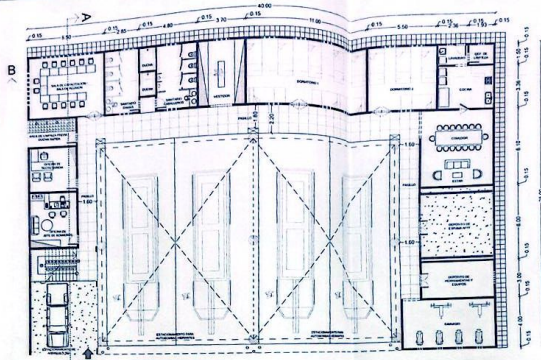
PLANTA BAJA BASE DE BOMBEROS SEI ASP Esc. 1/2000
