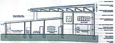
CORTE A-A BASE DE BOMBEROS SEI ASP Esc. 1/2000
