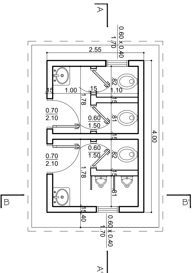
PLANTA ARQUITECTONICA
