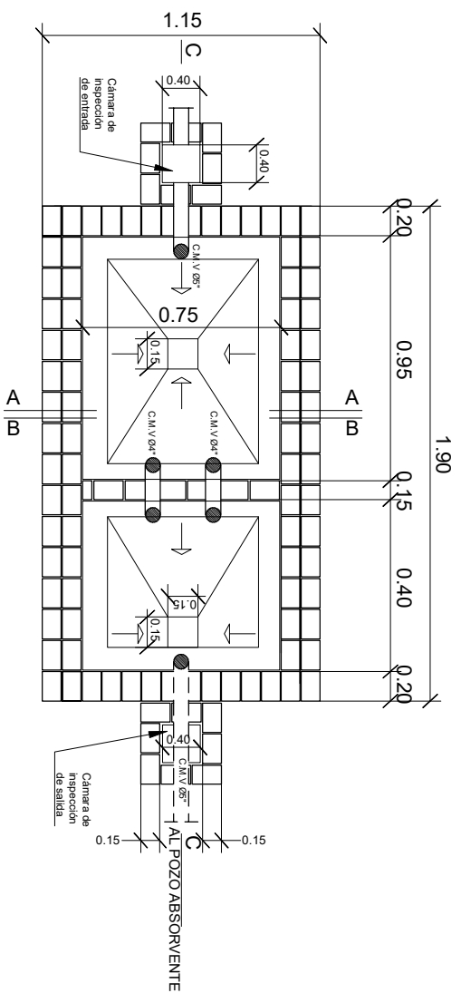
POZO CÁMARA SÉPTICA
