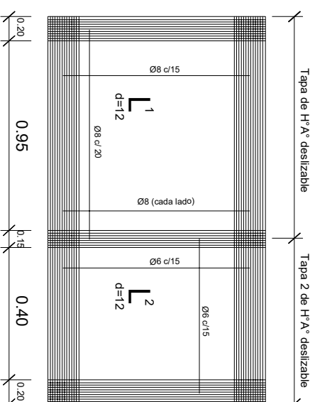
DETALLE DE LOSA CÁMARA SÉPTICA
