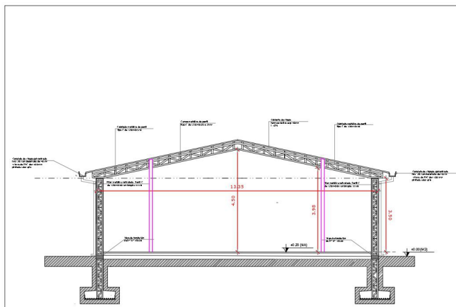
② CORTE TRANSVERSAL AA
