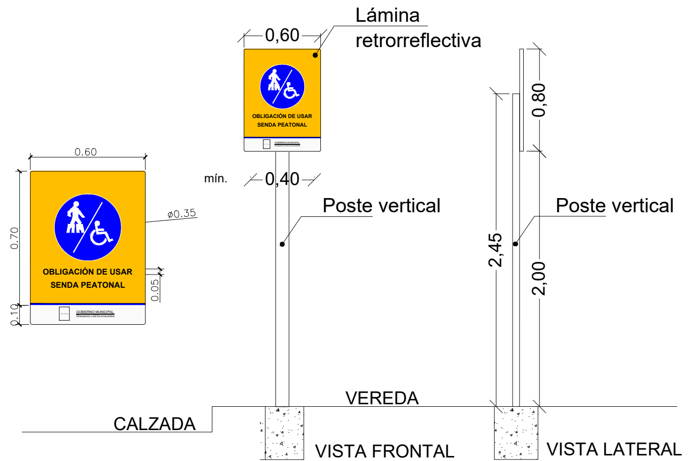
DETALLE SEÑALÉTICA EN CRUCE PEATONAL ESC.....1/50
