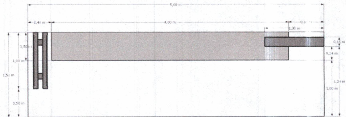
PLANTA ACOTADA
