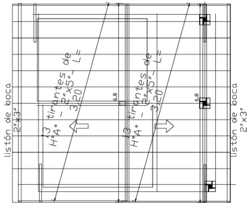
PLANTA ESTRUCTURA DE TECHO - CONSTRUCTIVA
