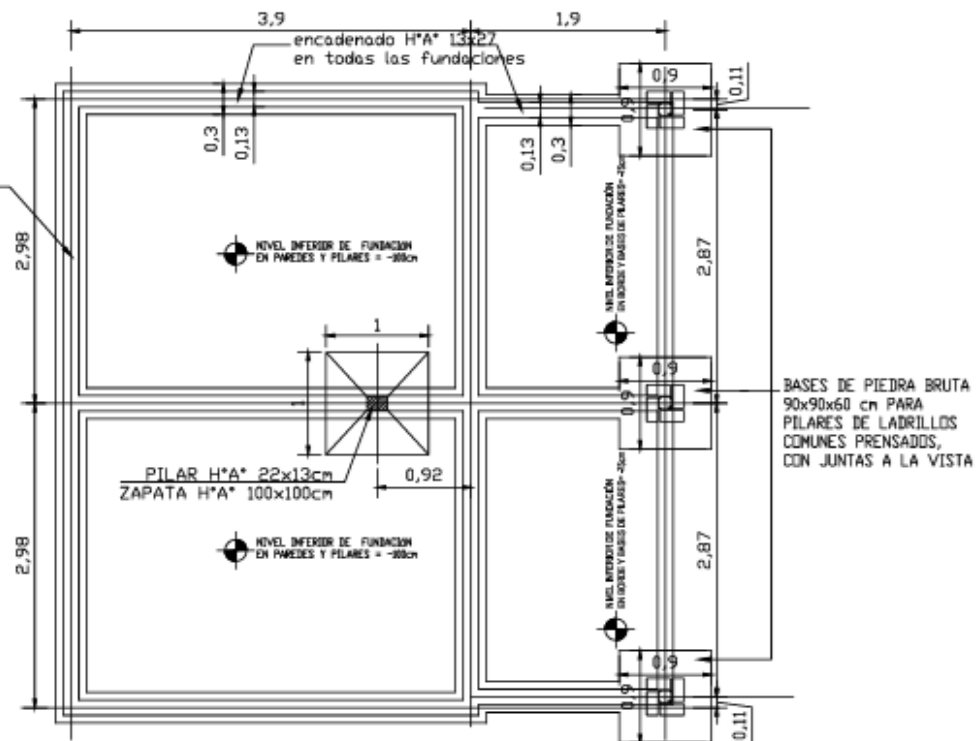
PLANTA DE FUNDACIONES
