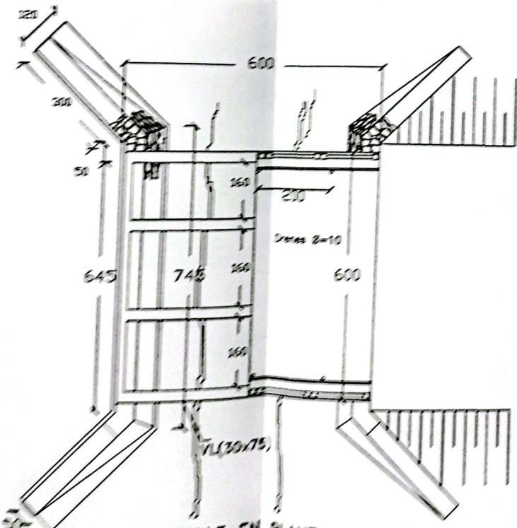
DETALLE EN PLANTA
