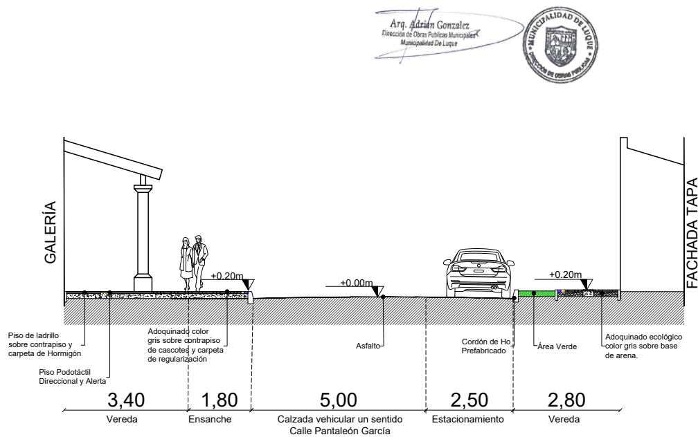
CORTE C-c. Ensanche y Vereda escala.....1/100
