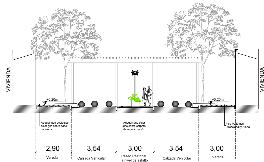
CORTE B-b. Paseo Peatonal escala.....1/100
