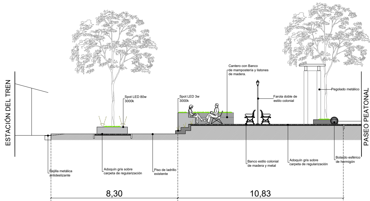
CORTE A-a. Revitalización de Plazoleta escala.....1/100
