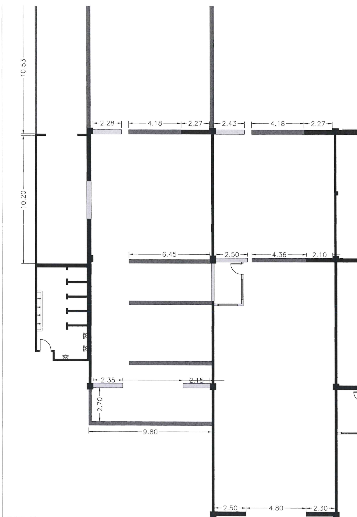
PLANTA ARQUITECTÓNICA ESC. 1/75
