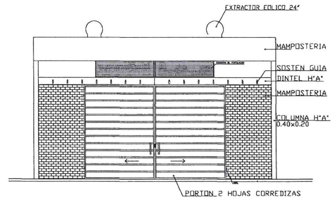
FACHADA ESC. 1/75
