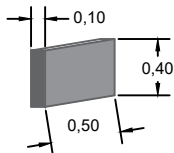
DETALLE DE CORDON NORMAL DE H*A (10X50X40)
