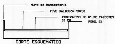
CORTE ESQUEMATICO
