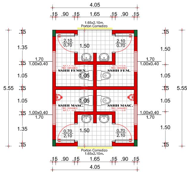
PLANTA ARQUITECTONICA Escala 1.50
