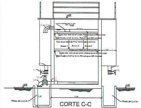
CORTE C-C
