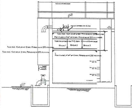
CORTE A-A
