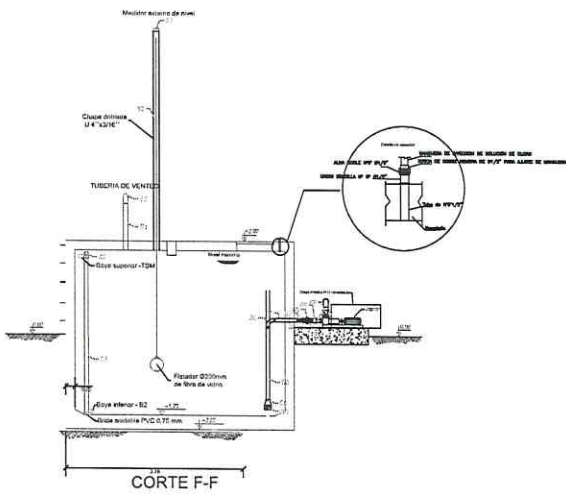
CORTE F-F
