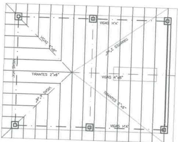
PLANTA DE TECHO
