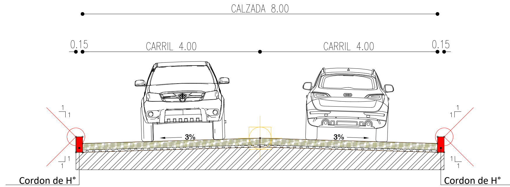
PAQUETE ESTRUCTURAL DEL PAVIMENTO
