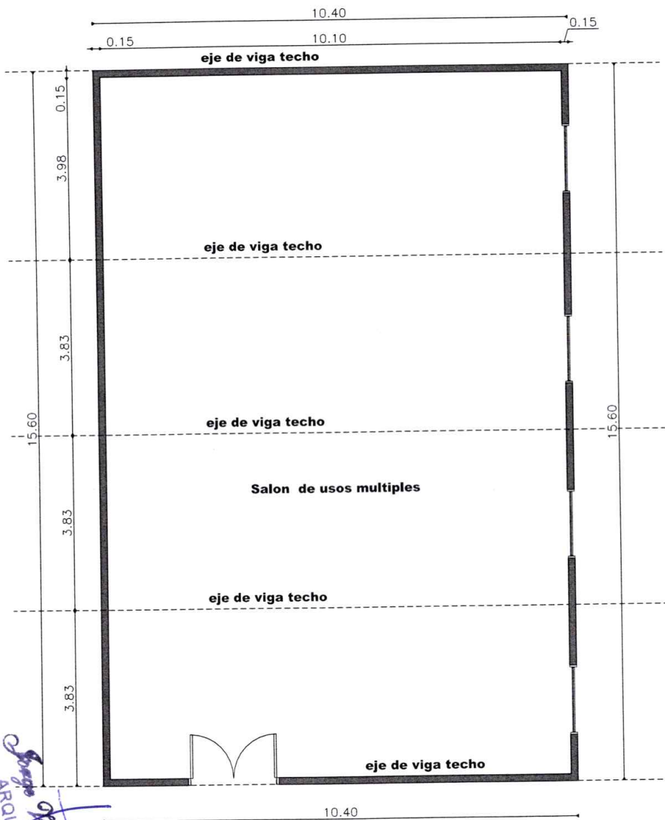
PLANO ACOTADO ESC. 1/75
