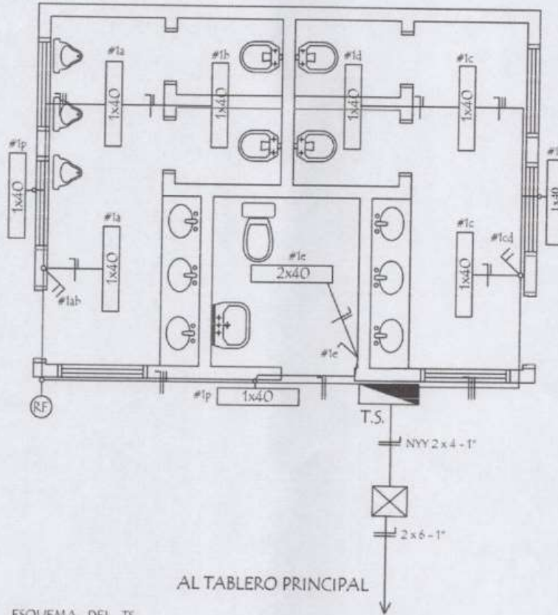
ESQUEMA DEL TS AL TABLERO GENERAL
