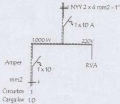
ESQUEMA DEL TS AL TABLERO GENERAL
