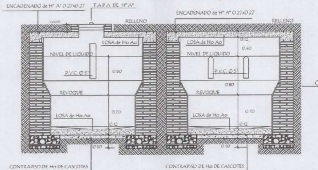
Corte BB
