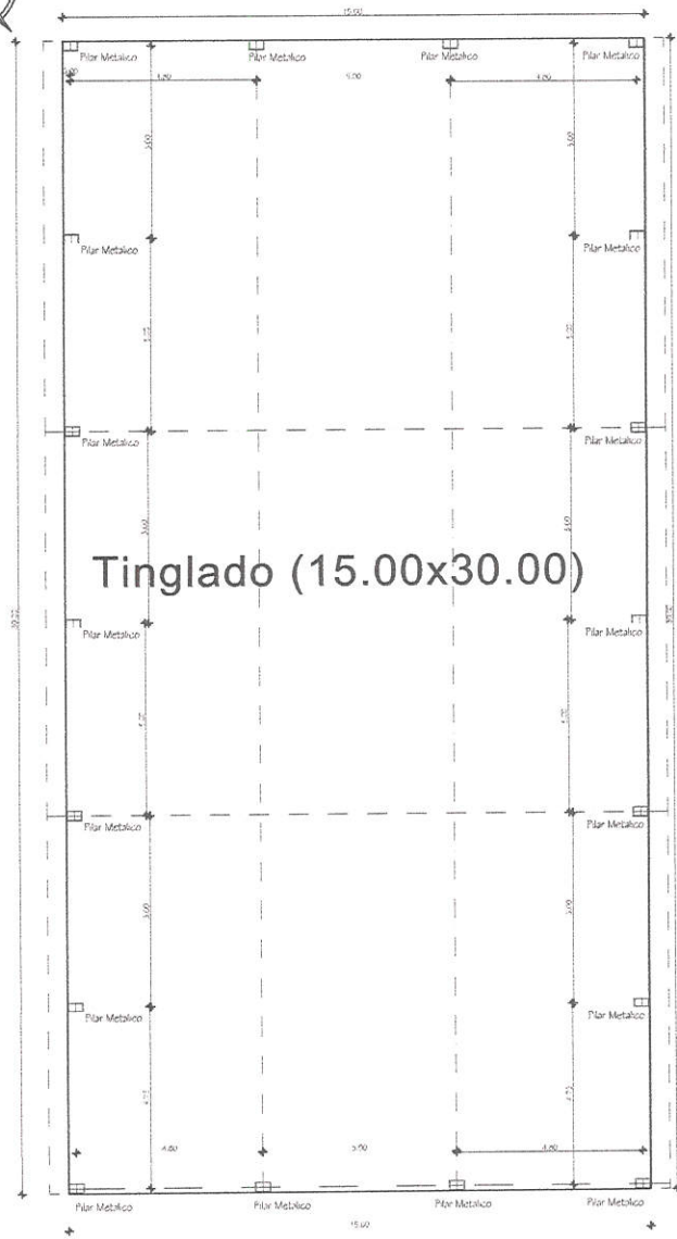
Planta Arquitectonica
