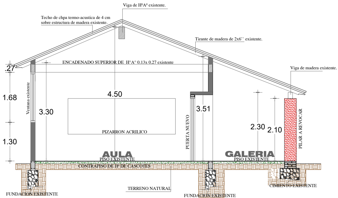
CORTE A-A (Proyectado)
