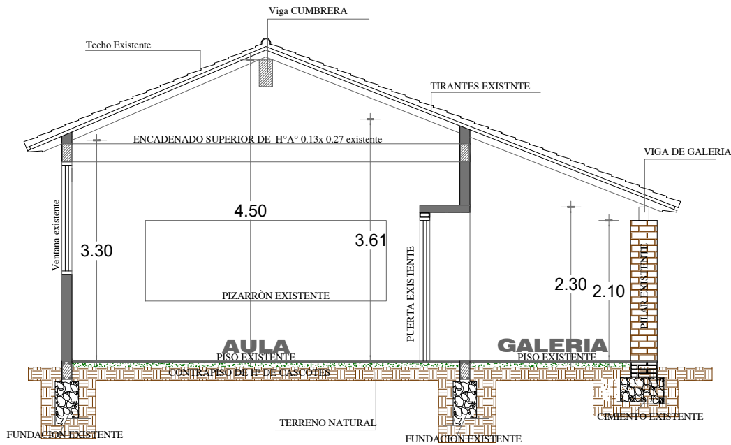
CORTE A-A (Existente)
