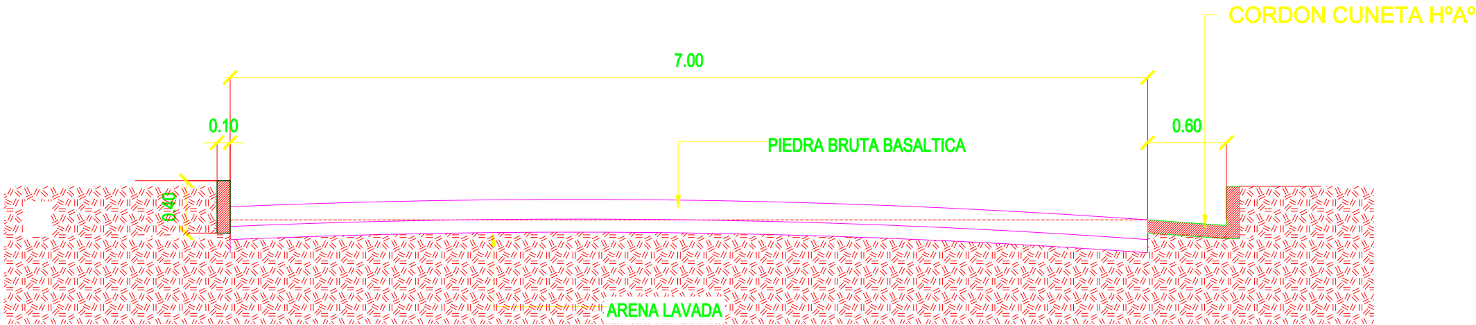
CORTE TRANSVERSAL
