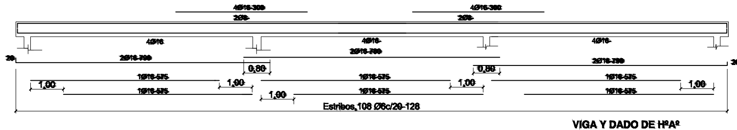
VIGA Y DADO DE HºAº
