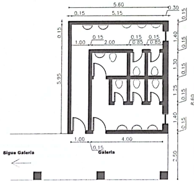
PLANTA SANITARIO ESC. 1/75
