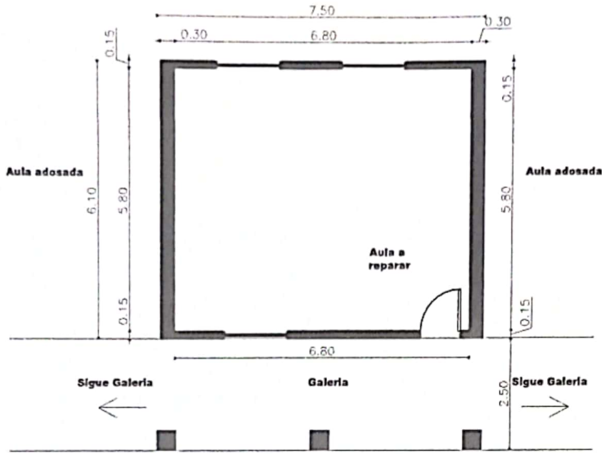
PLANTA AULA ESC. 1/75
