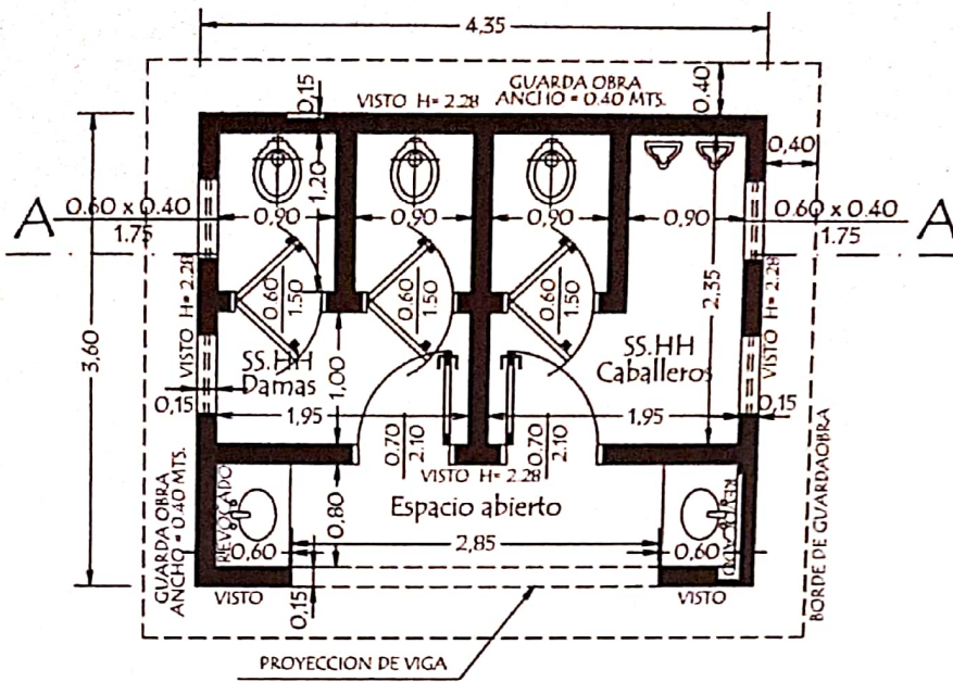
PLANTA CONSTRUCTIVA
