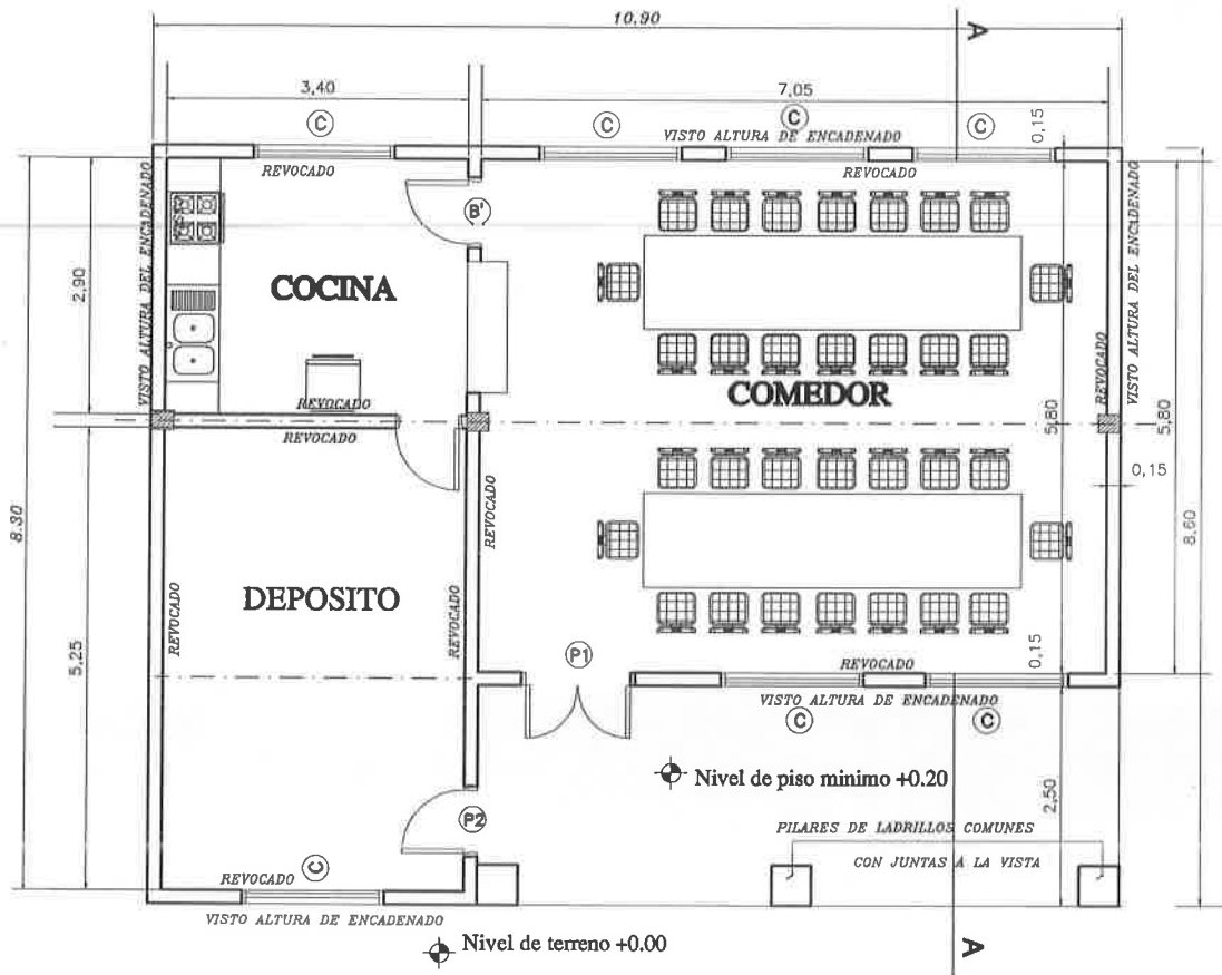
PLANTA ----- ESC. 1/75
