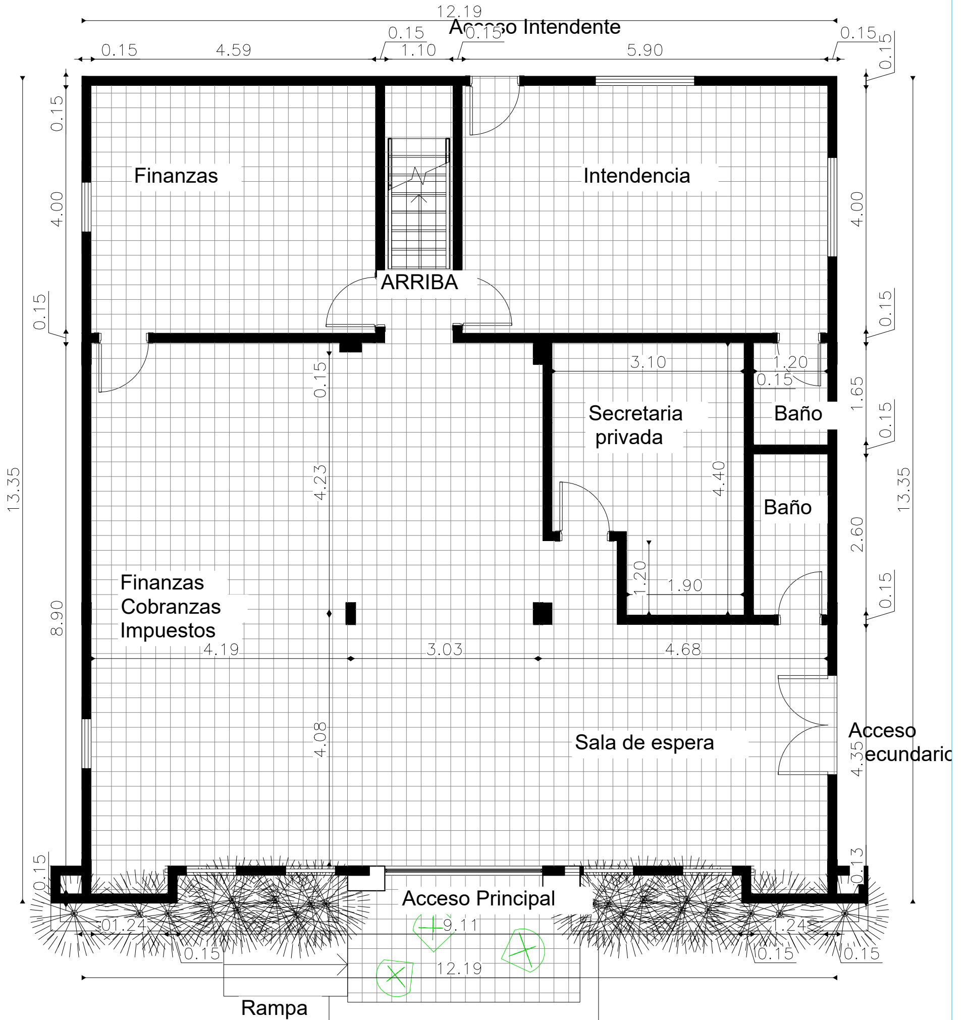
Planta Baja Acotada ESC. 1/75
