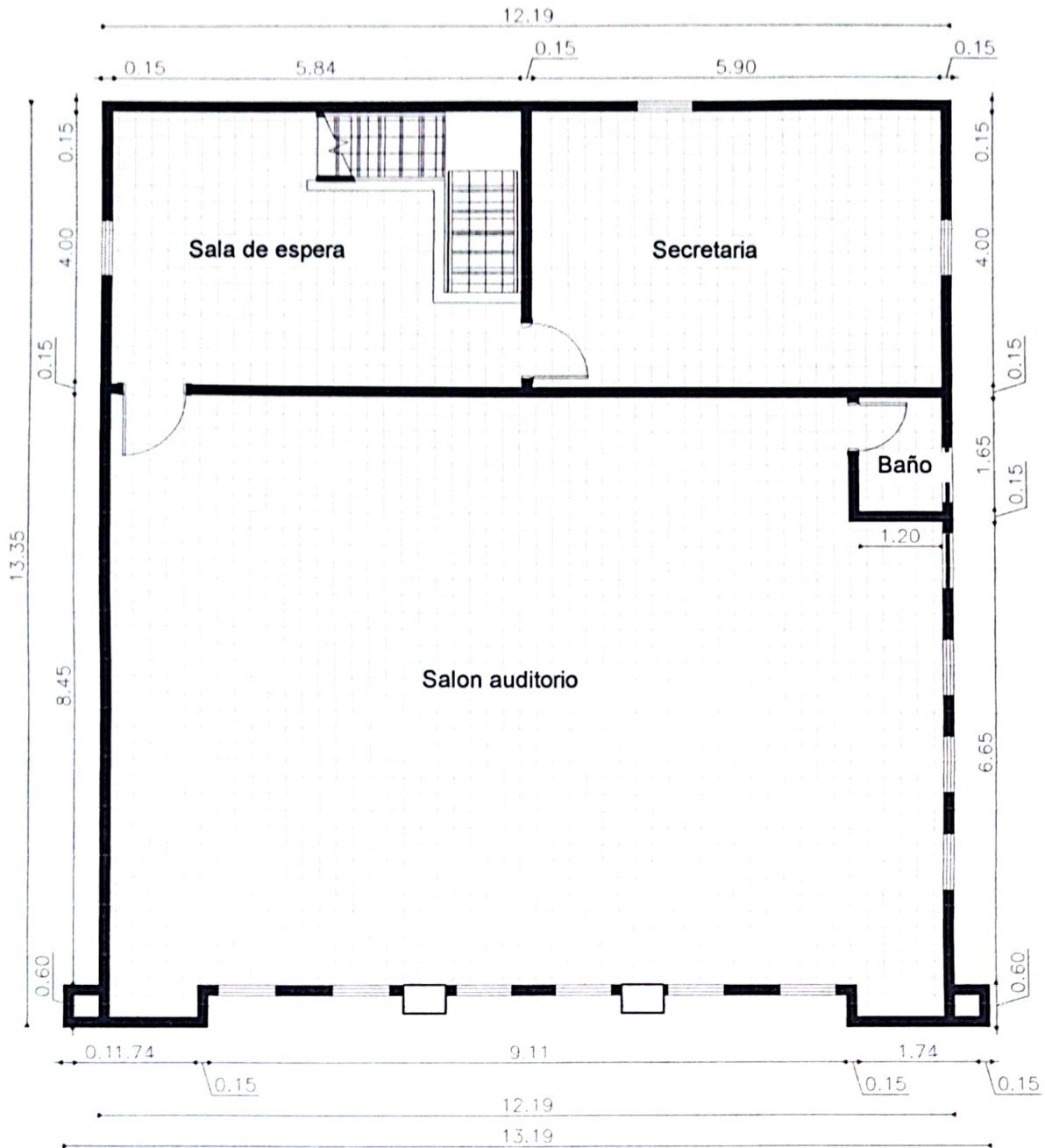
Planta Alta Acotada ESC. 1/75
