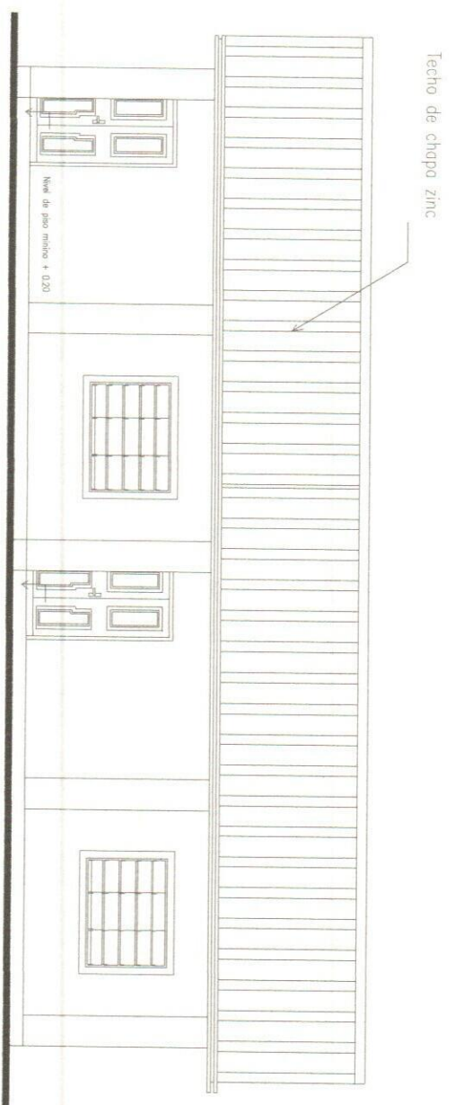
FACHADA FRONTAL
